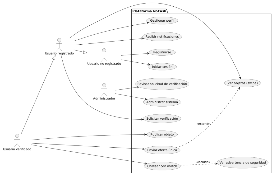
Ilustración 1. Diagrama de caso de uso NoCash
